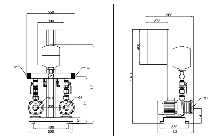
DIMENSÕES BOOSTER MCH2-R
