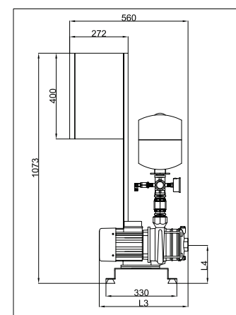
DIMENSÕES BOOSTER MCH-1
