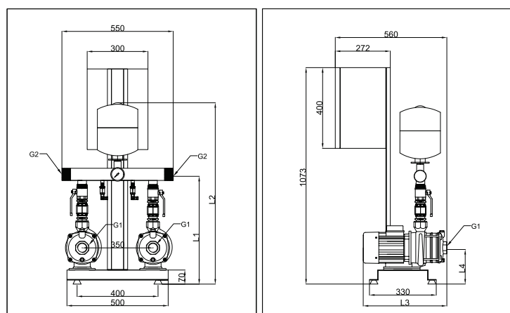
DIMENSÕES BOOSTER MCH-2S
