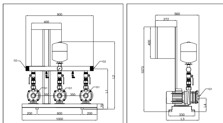
DIMENSÕES BOOSTER MCH-3S
