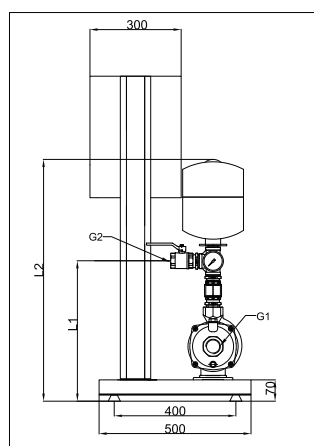
DIMENSÕES BOOSTER MCH-1
